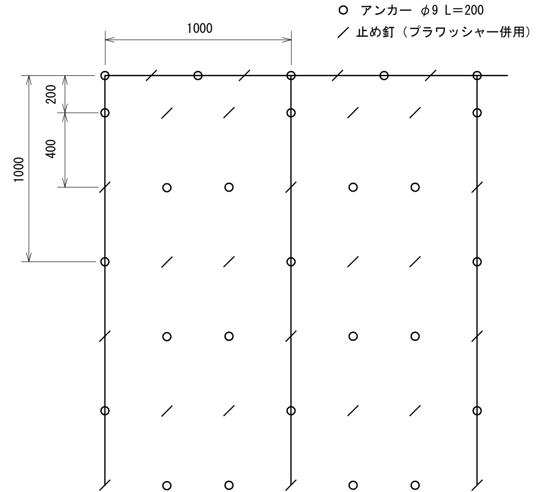
標準展開図
