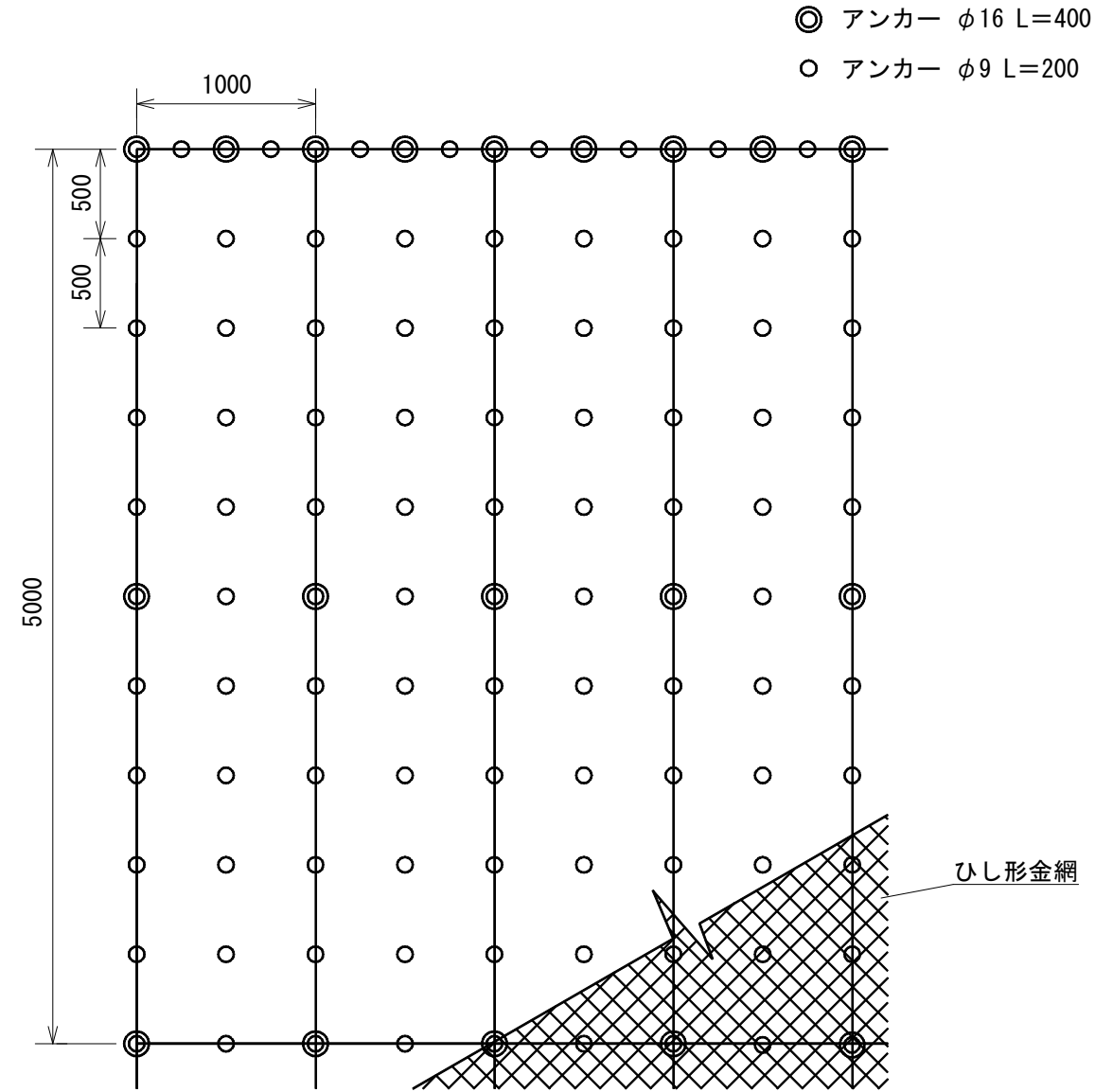
標準展開図
