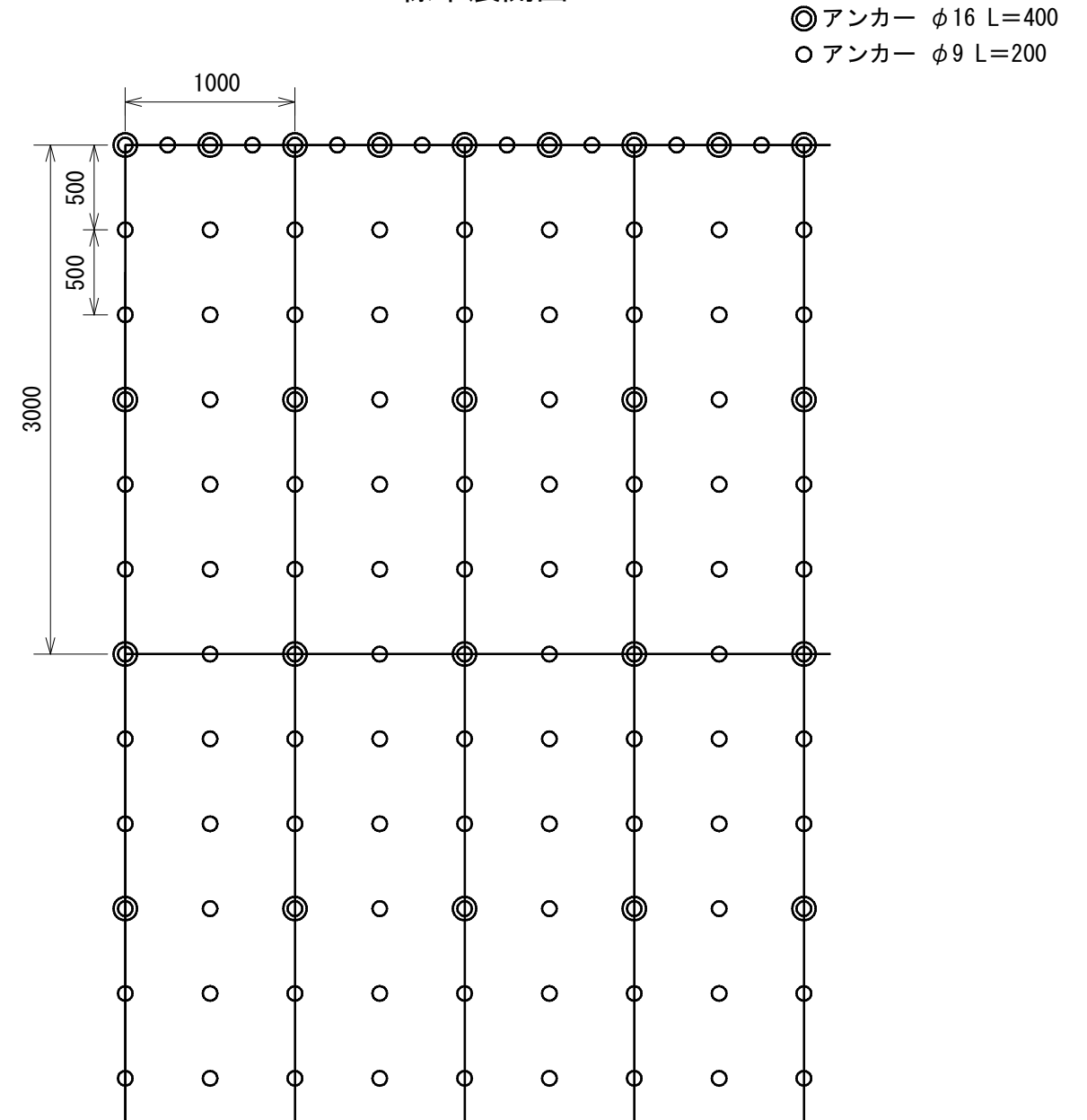
標準展開図
